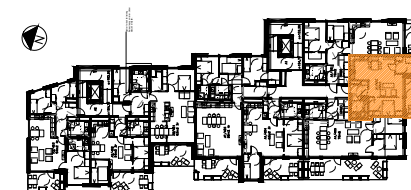
PLAN 4 ETASJE
