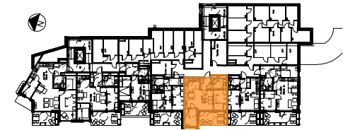
PLAN 2 ETASJE
